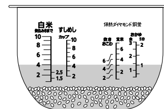
(白米4カップの場合) 図の内釜は1.8Lタイプです。
